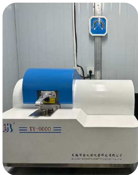
光谱分析 Spectral Analysis
